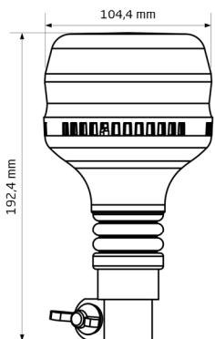
Aufsteckversion
